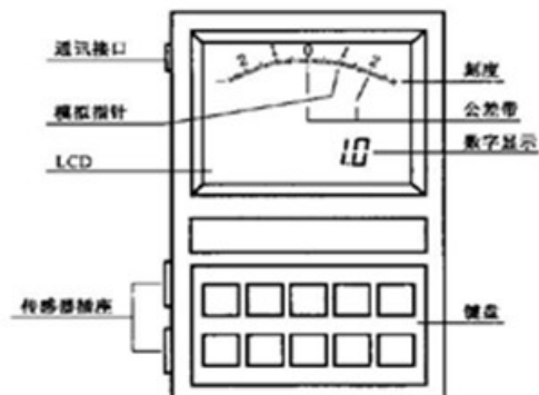
图 2 带模拟表显示的数显电感测微仪的型式示意图
