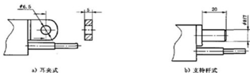
图 5 旁向式传感器装夹部位的型式示意图
