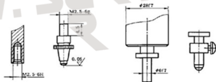
图 6 轴向式传感器测头的连接尺寸示意图
